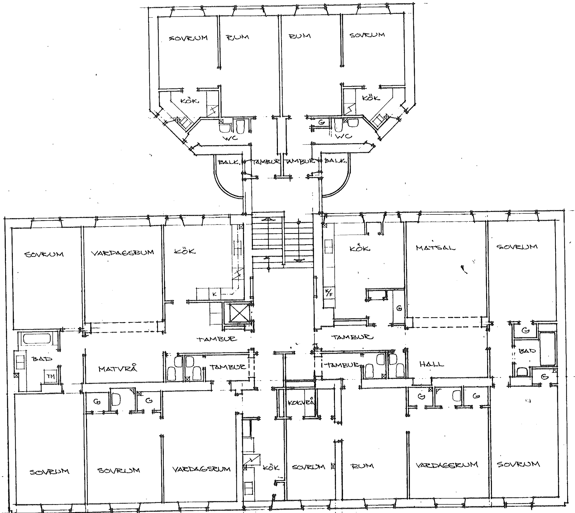
PLAN 1TR
